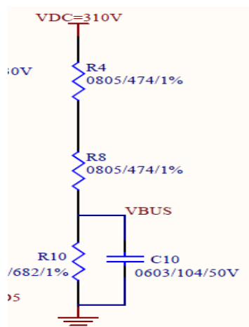
图 3-3 分压比电路
