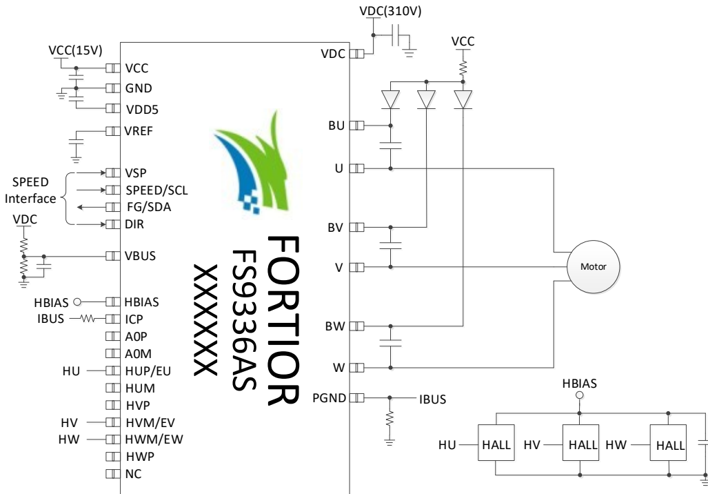
图 1-2 有感 3 HALL IC 输入模式
