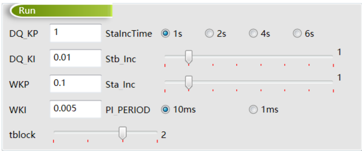
图 3-9 运行参数
