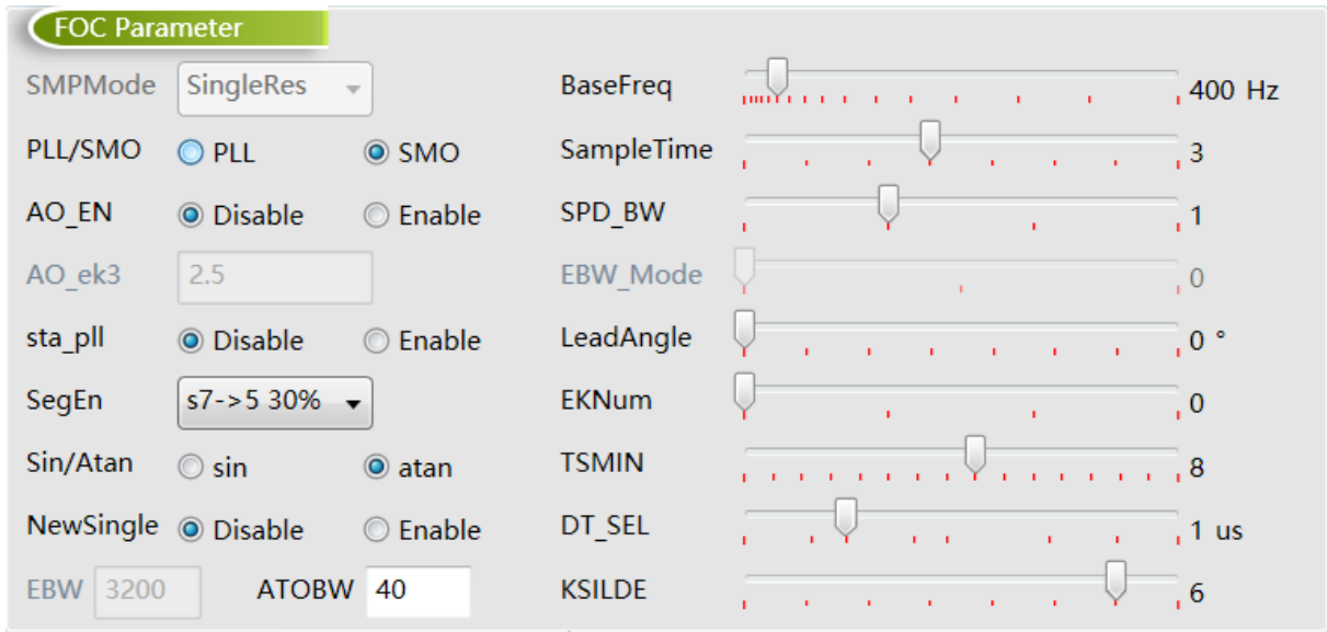
图 3-4 FOC 参数
