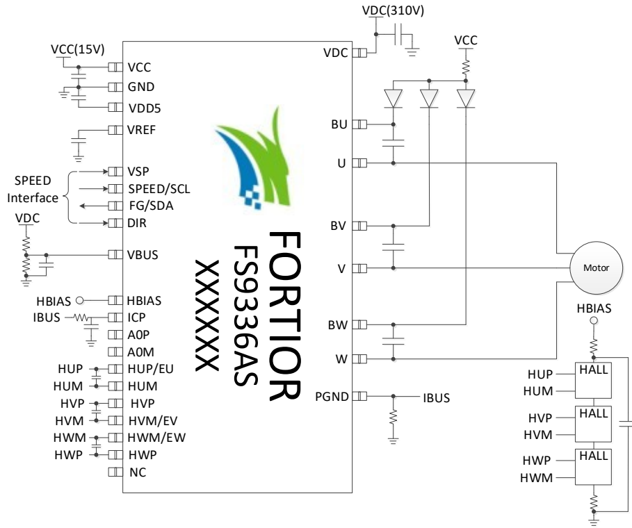
图 1-1 有感 3 HALL 差分输入模式
