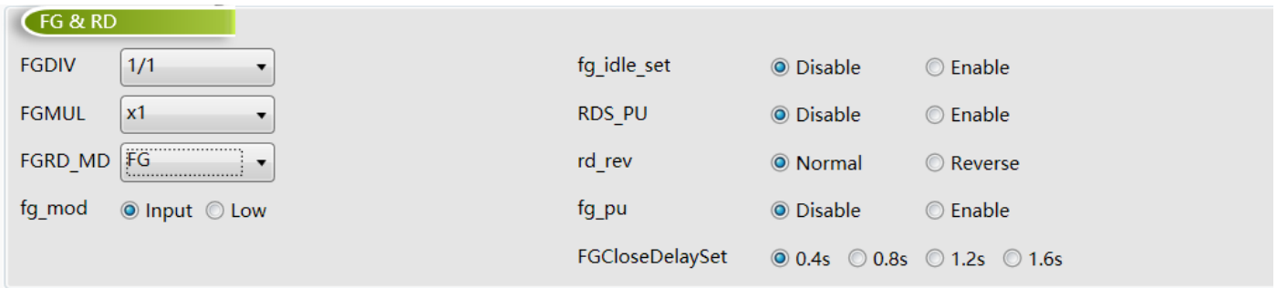
图 3-12 调速&FG/RD
