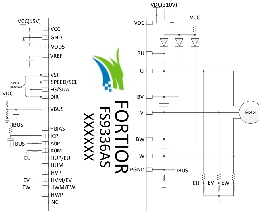
图 1-3 无感单电阻差分采样 FOC 模式
