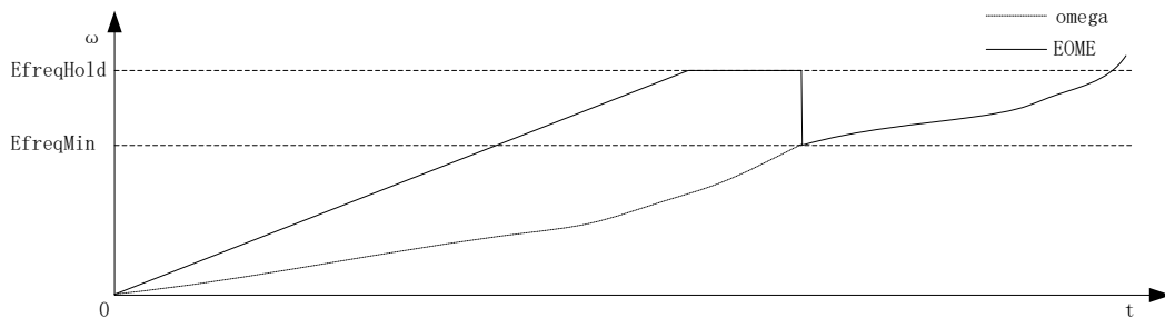
图 3-6 启动过程图
