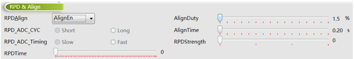
图 3-10 转子位置检测&预定位
