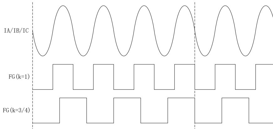
图 3-13 k = 1 和 k = 3/4 的 FG 输出图
