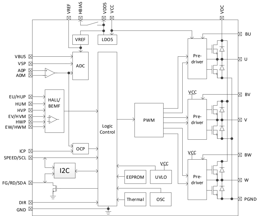
图 1-4 FS93XXAS 功能框图
