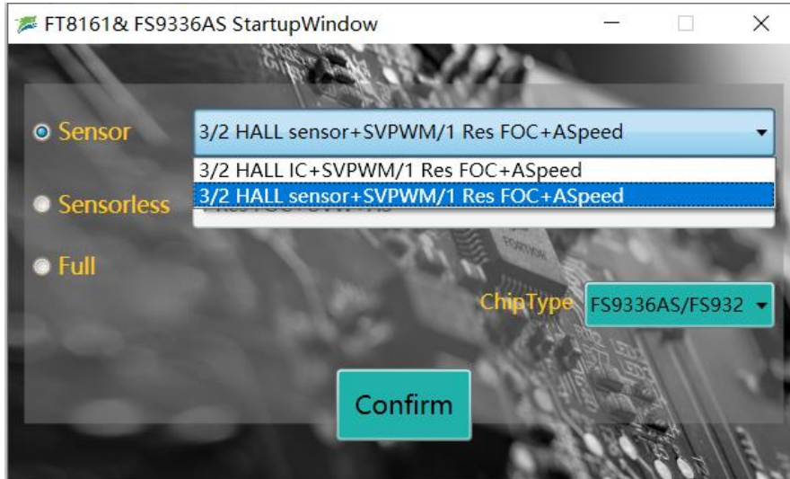
图 2-3 上位机界面
