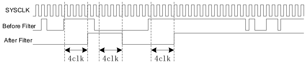
16-4 滤波模块时序图
