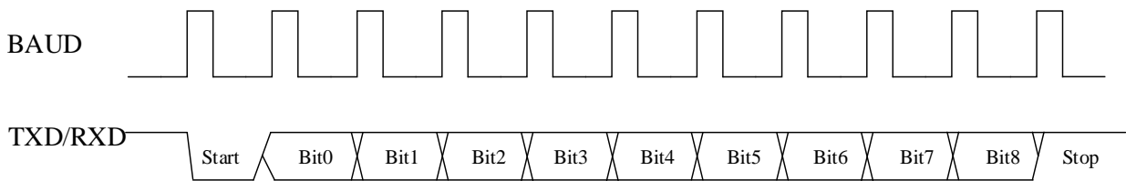
图 10-2 UART 通信时序图
