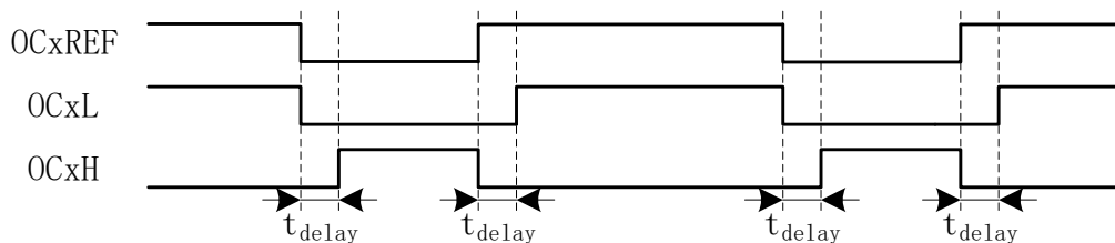
图 18-4 带死区插入的互补输出
