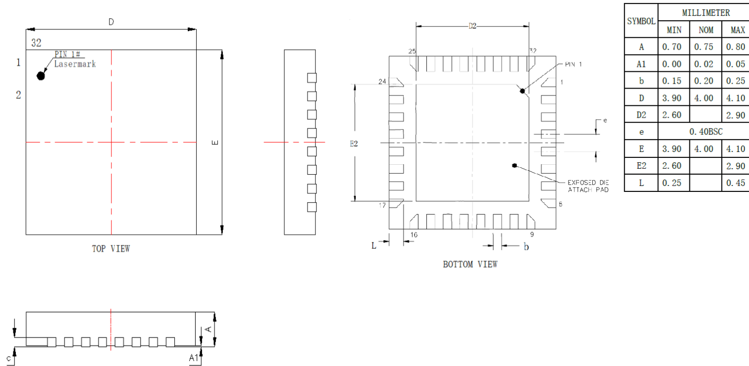
图 3-1 QFN32_4X4 封装尺寸图
