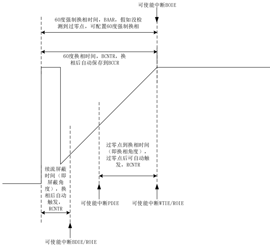
图 14-6 BLDC 的工作原理
