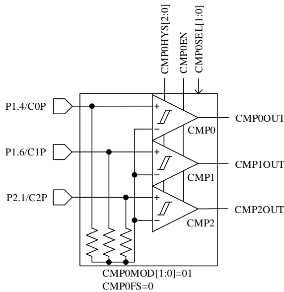
图 28-9 有内置电阻三比较器模式，无功能转移
