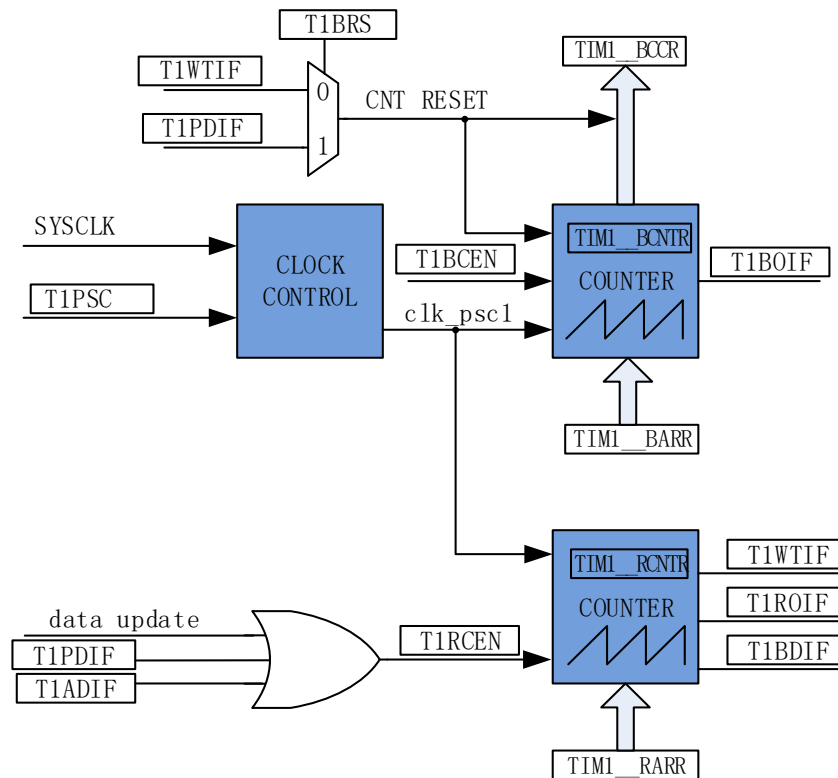
图 14-2 时基单元
