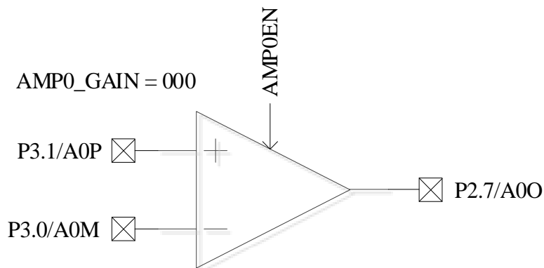
图 27-2 母线电流运放 AMP0
