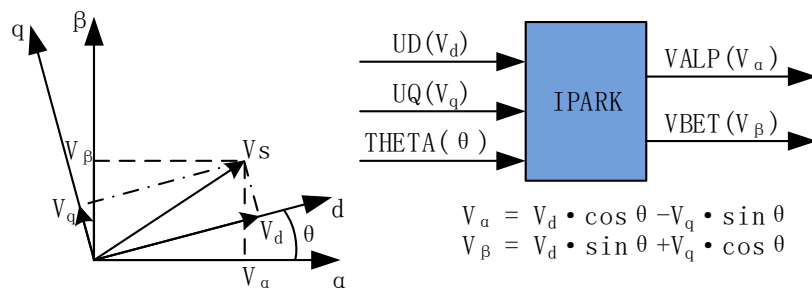
图 13-2 Park 逆变换
