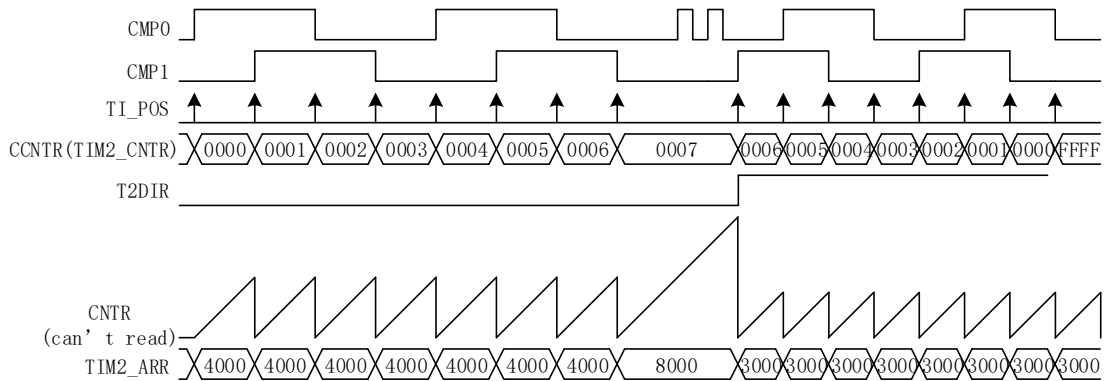
图 15-10 RSD 模式时序图
