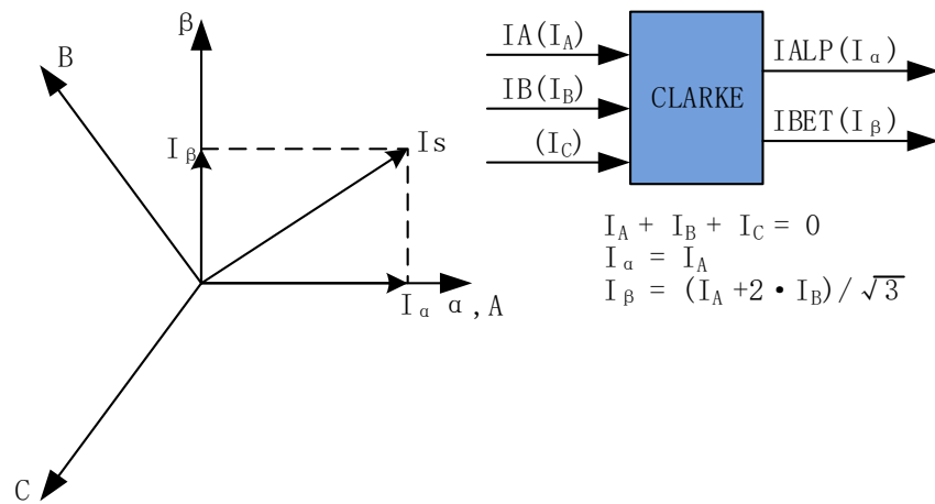
图 13-4 Clarke 变换
