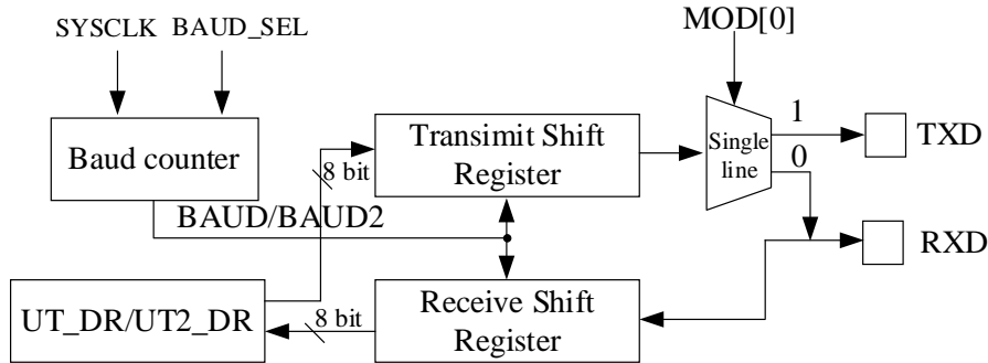
图 10-1 UART 通信模块构造框图
