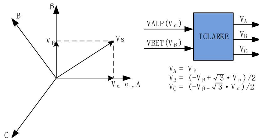
图 13-3 Clarke 逆变换
