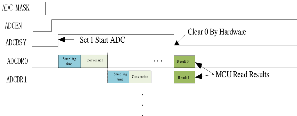
图 22-3 ADC 顺序采样时序图
