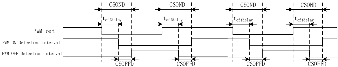
图 14-5 采样区间图
