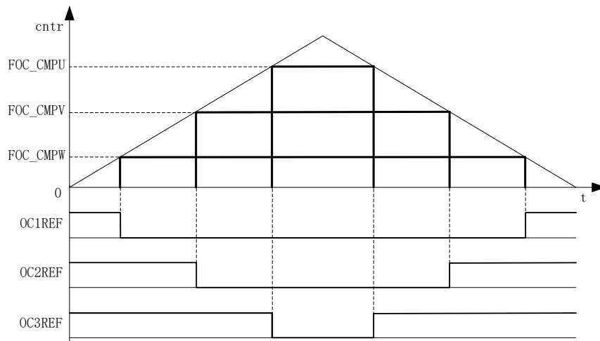
图 18-3 PWM 生成图
