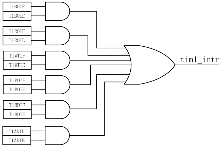
图 14-10 Timer1 中断源
