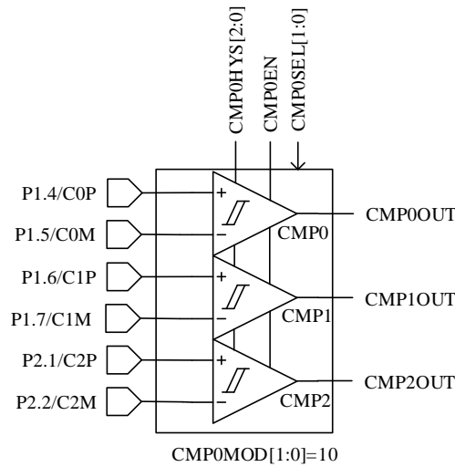
图 28-11 择差分三比较器模式
