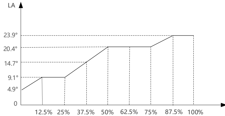
图 5-6 提前角曲线
