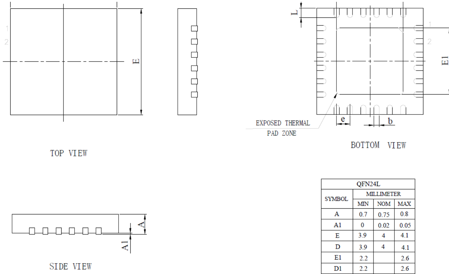
图 2-1 FT8132Q QFN24_4X4 封装尺寸图
