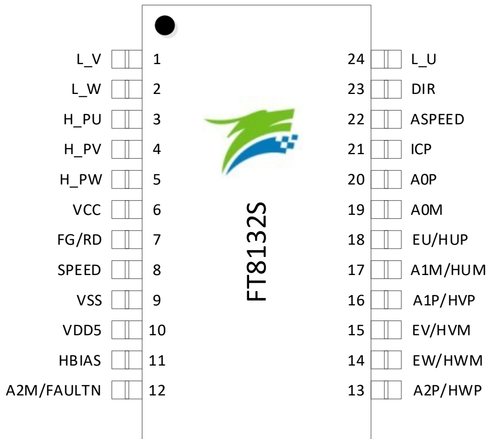
图 1-6 FT8132 SSOP24 引脚图
