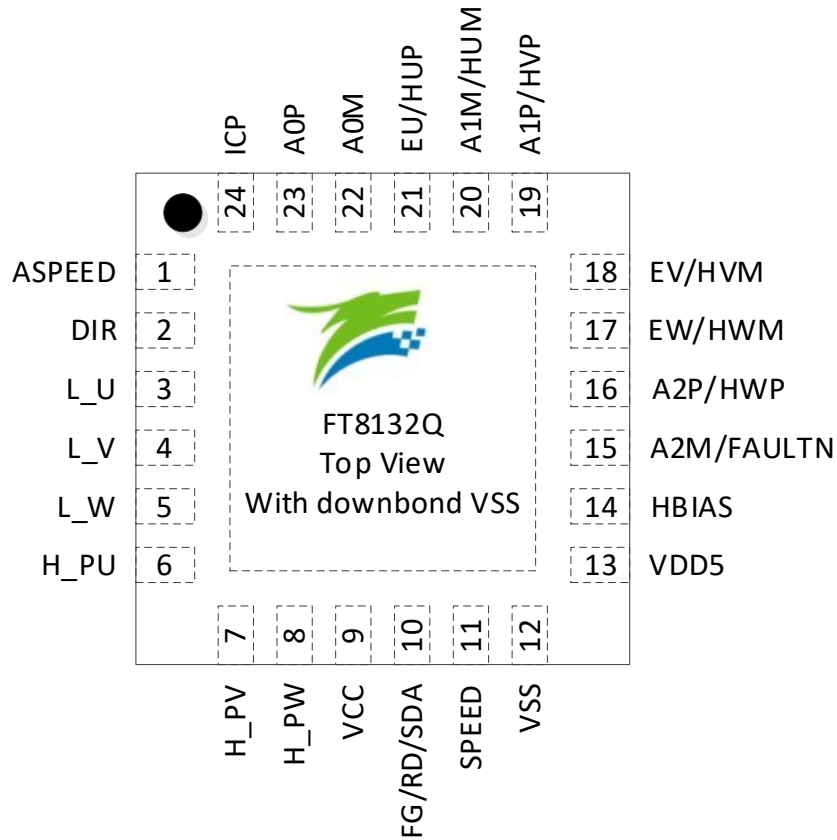
图 1-5 FT8132 QFN24 引脚图
