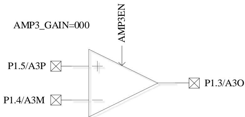
图 30-11 AMP3 输入输出相关端口
