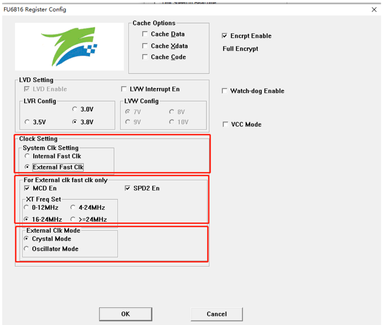
图 23-6 FU6816L 系统时钟配置
