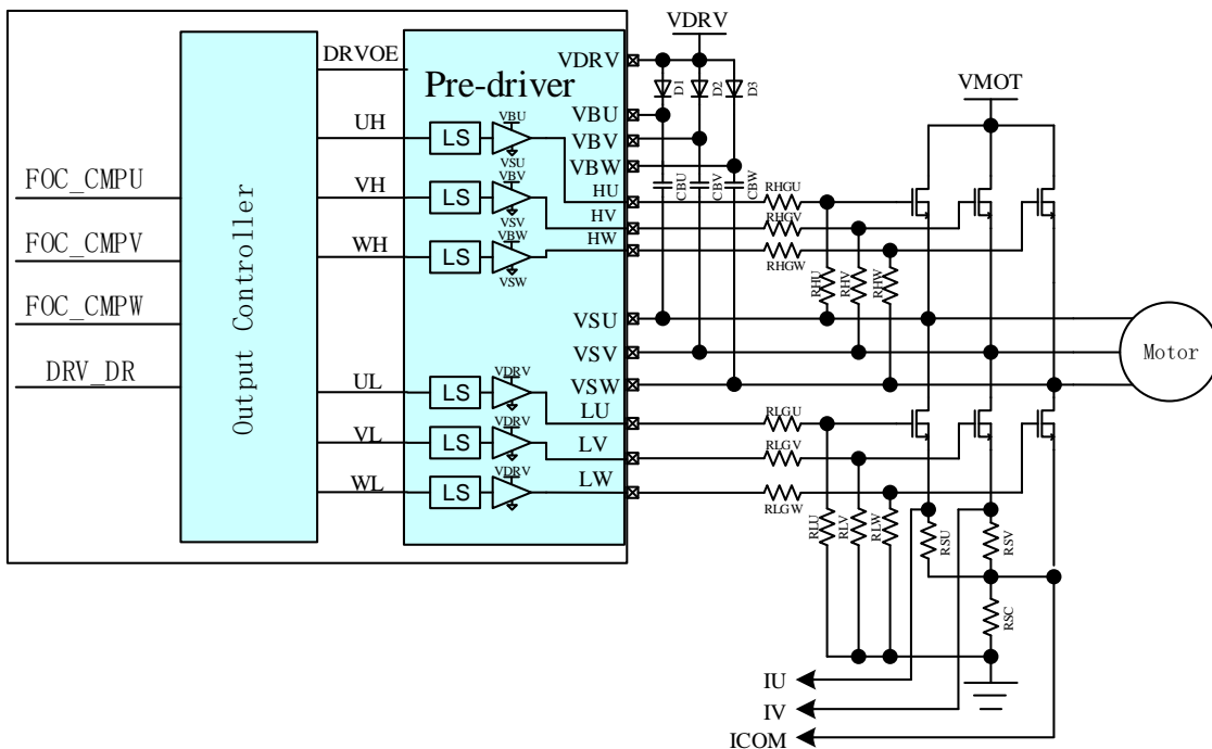
图 19-2 FU6866Q Driver 模块框图
