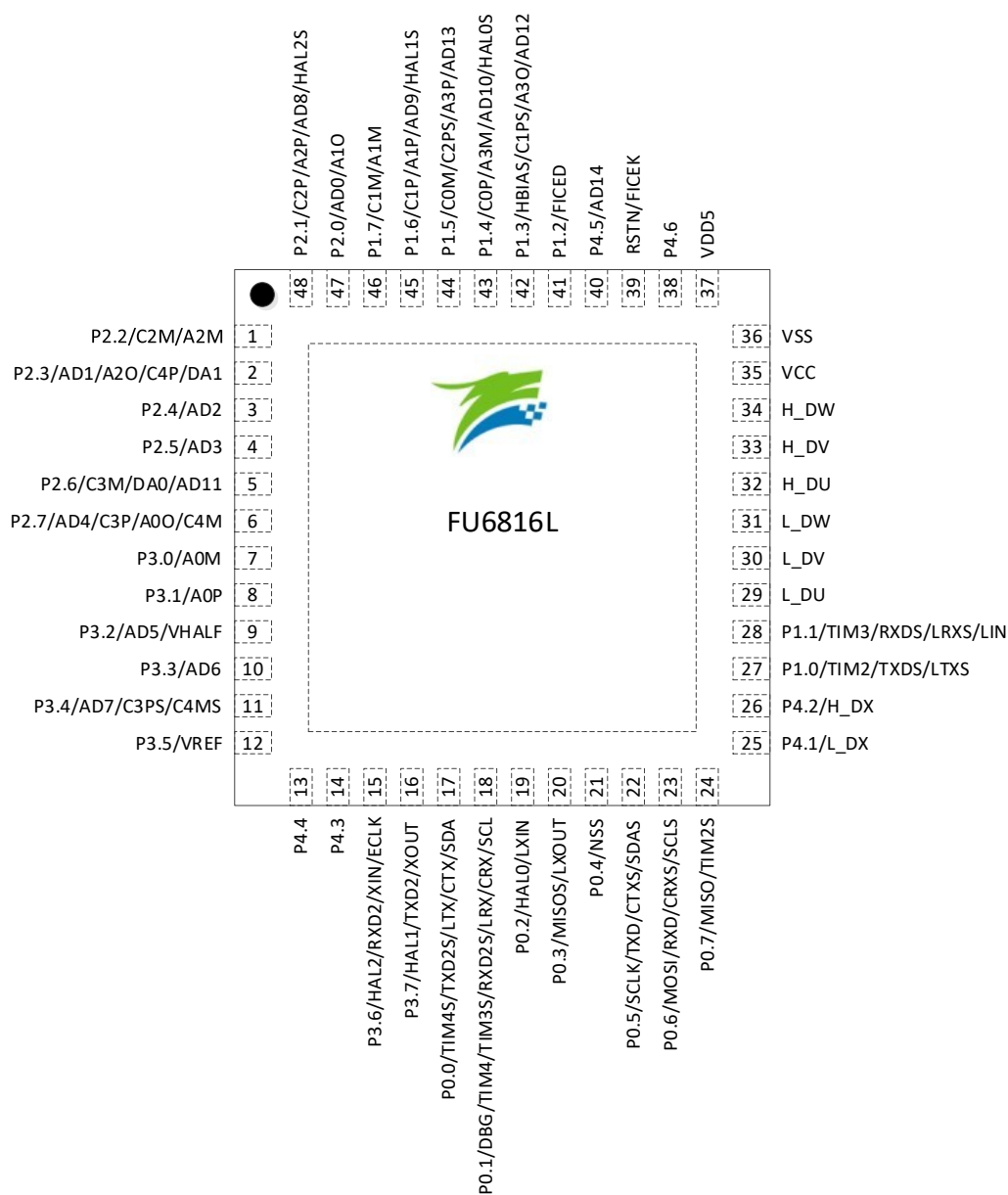
图 2-1 FU6816L LQFP48 引脚图
