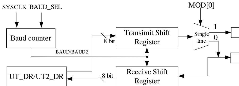
图 10-1 UART 通信模块构造框图
