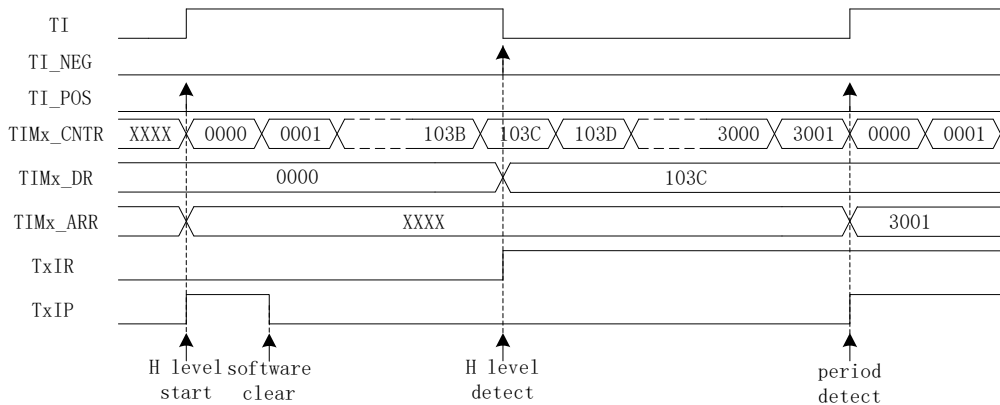
图 17-6 输入捕获模式(TIMx_CR0[TxOCM] = 0)时序图
