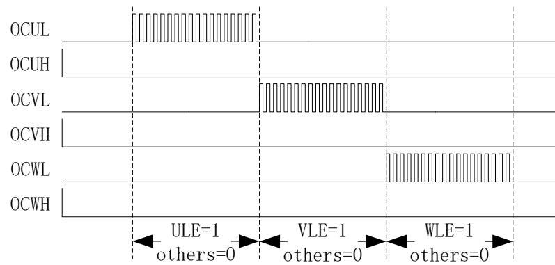
图 19-7 预充电波形图
