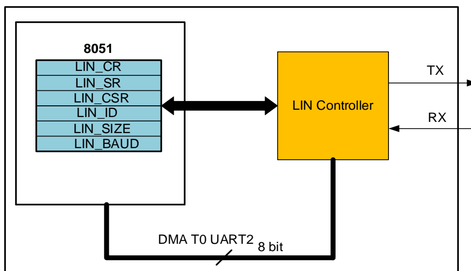
图 11-1 LIN 框图
