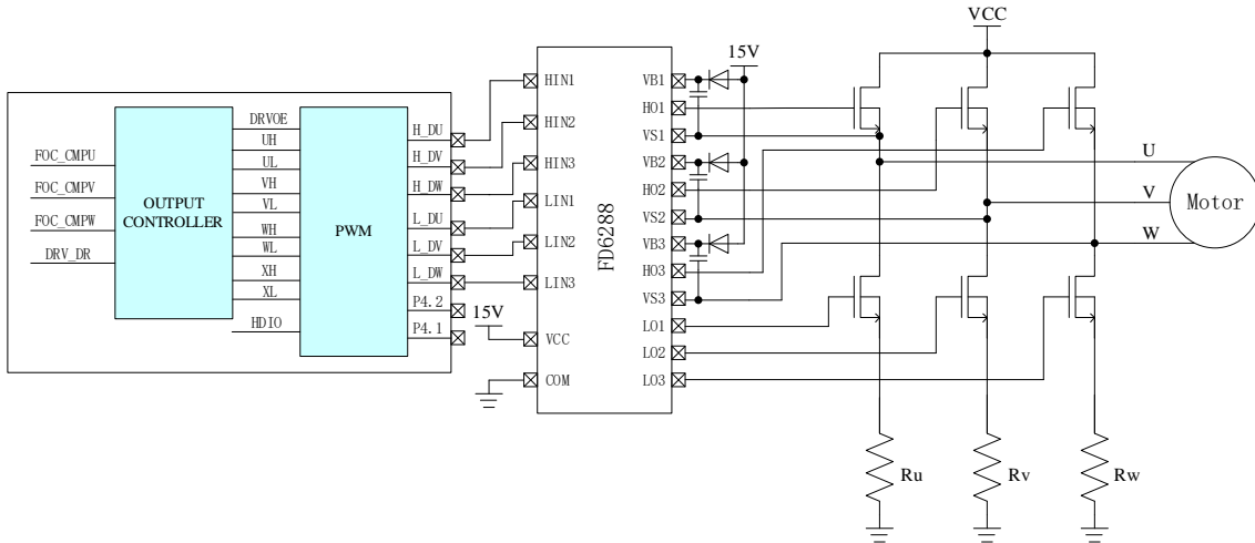
图 19-1 FU6816L Driver 模块框图
