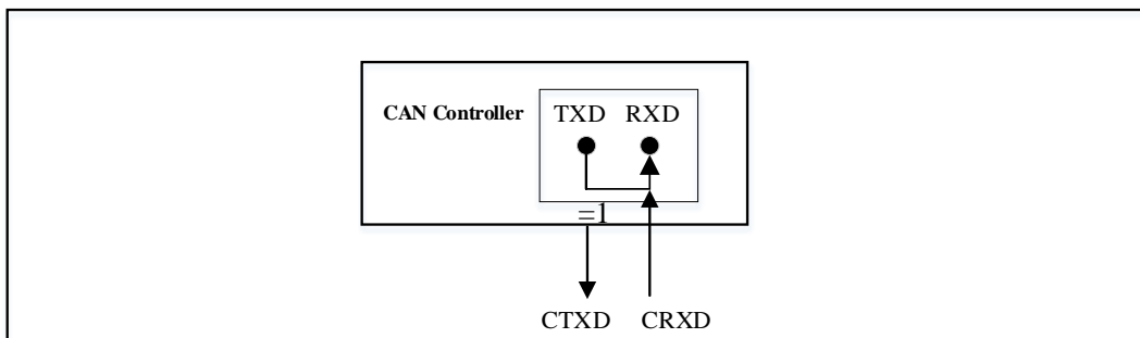
图 12-12 监听模式
