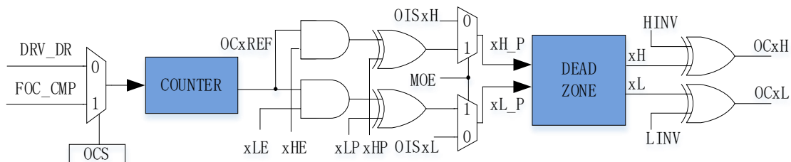
图 19-3 输出控制模块前级框图
