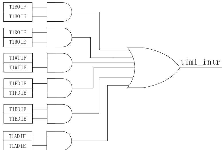
图 15-10 Timer1 中断源
