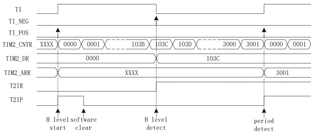
图 16-6 输入捕获模式(TIM2_CR0[T2CES] = 0)时序图
