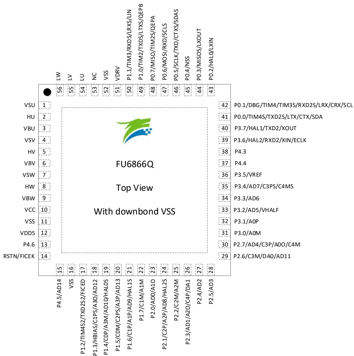
图 2-2 FU6866Q QFN56 引脚图
