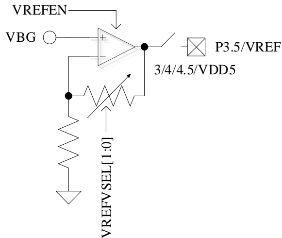
图 28-1 VREF 模块输入输出端口
