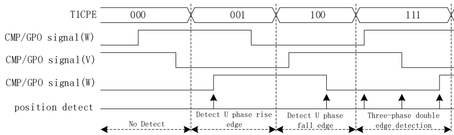
图 15-6 位置检测时序图
