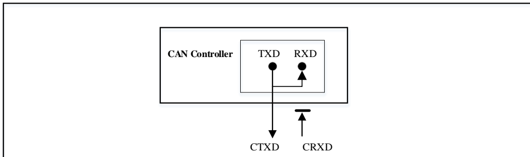
图 12-11 自测模式
