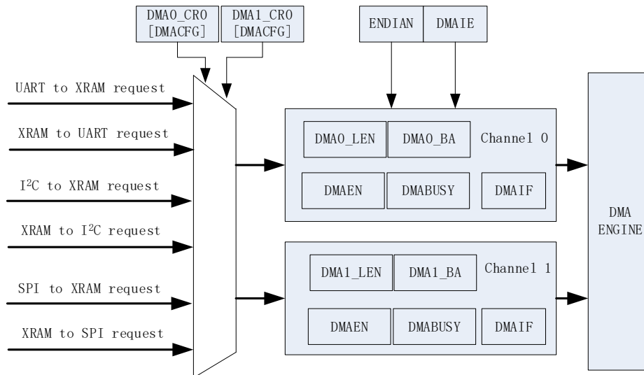
图 27-1 DMA 功能框图
