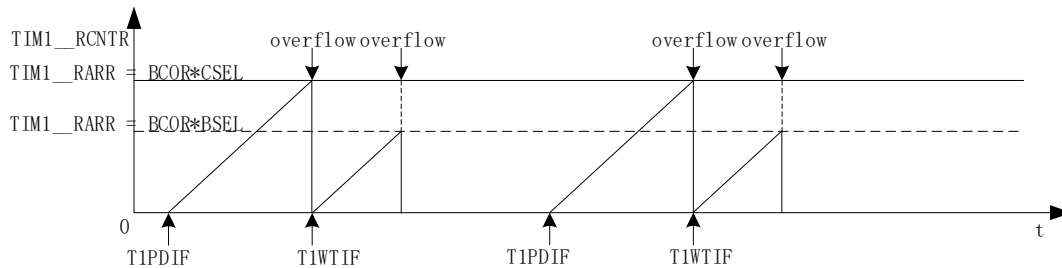
图 15-4 重载计数器计数波形图
