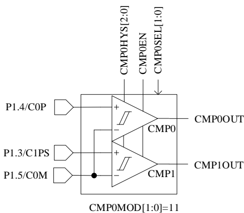
图 31-12 比较器模式
