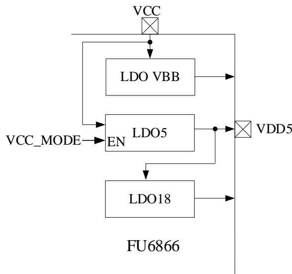
图 32-3 FU6866Q 电源模块功能框图
