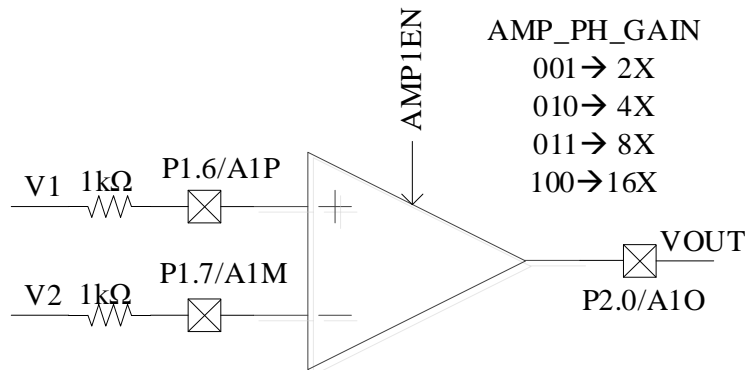
图 27-7 AMP1 工作在 PGA 差分输入模式
