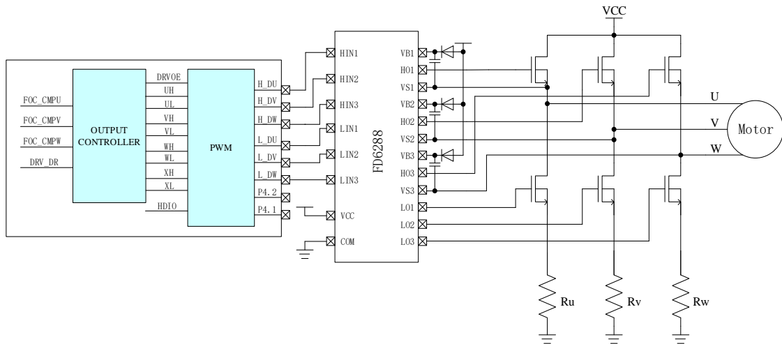
图 18-1 FU6815Q1 Driver 模块框图
