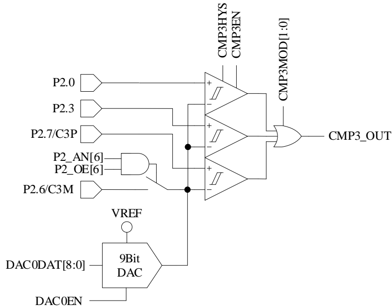
图 28-4 三比较器输入模式
