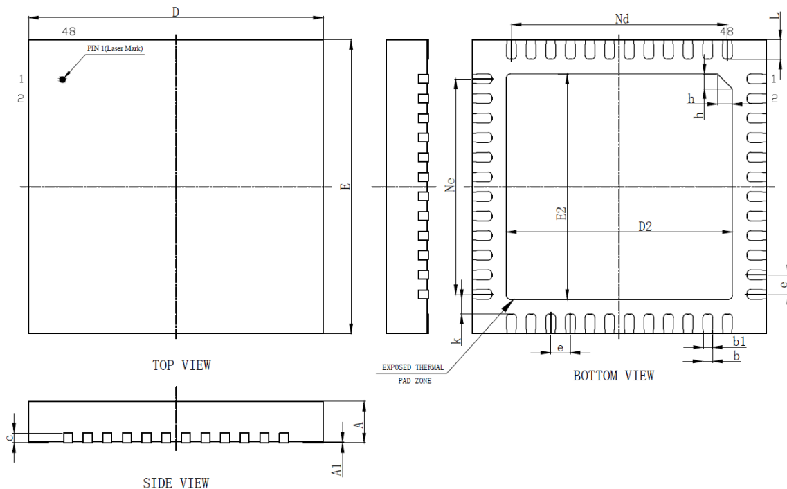
图 3-1 QFN48_6X6 封装尺寸图
