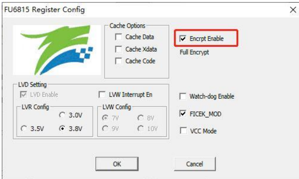
图 33-2 代码保护 全保护模式
