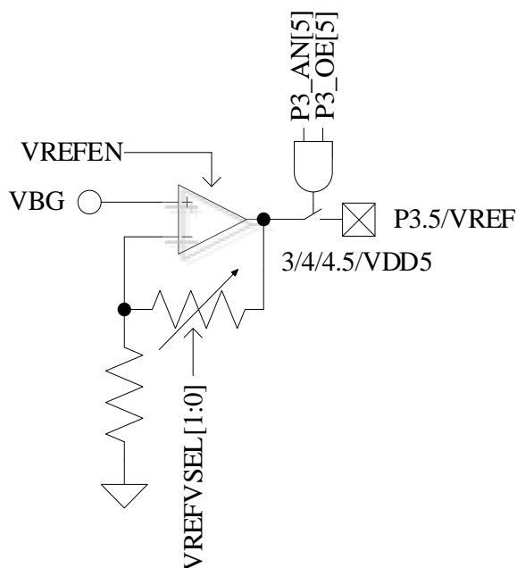
图 25-1 VREF 模块输入输出端口
