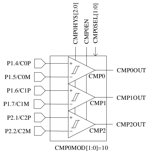
图 28-12 差分三比较器模式
