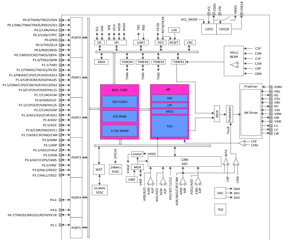
图 1-2 FU6865Q1 功能框图
