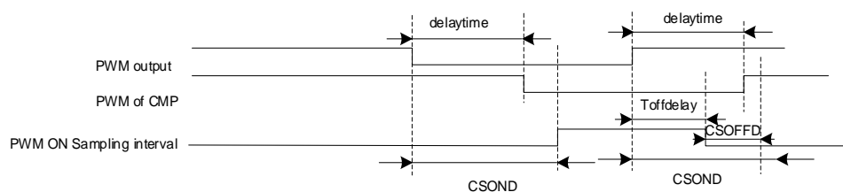
图 28-15 PWM OFF 采样模式
