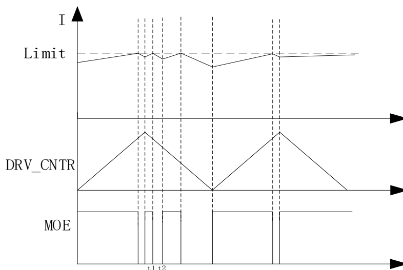
图 28-6 EVT_FILTER[MOEMD] = 11, 逐波限流波形( t_2 - t_1 = 5\mu\text{s} )
