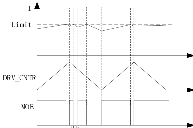
图 28-5 EVT_FILT[MOEMD] = 10 ，逐波限流波形( t_2 - t_1 = 10\mu\text{s} )
