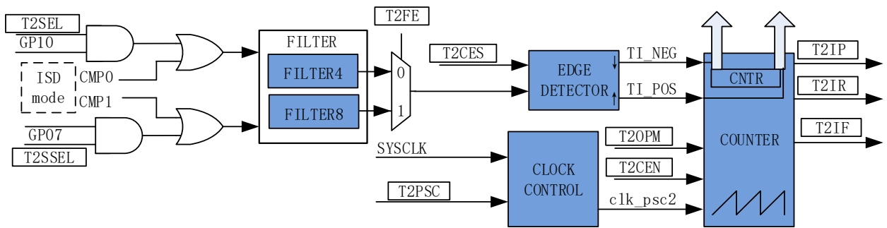
图 15-5 输入捕获模式原理框图
