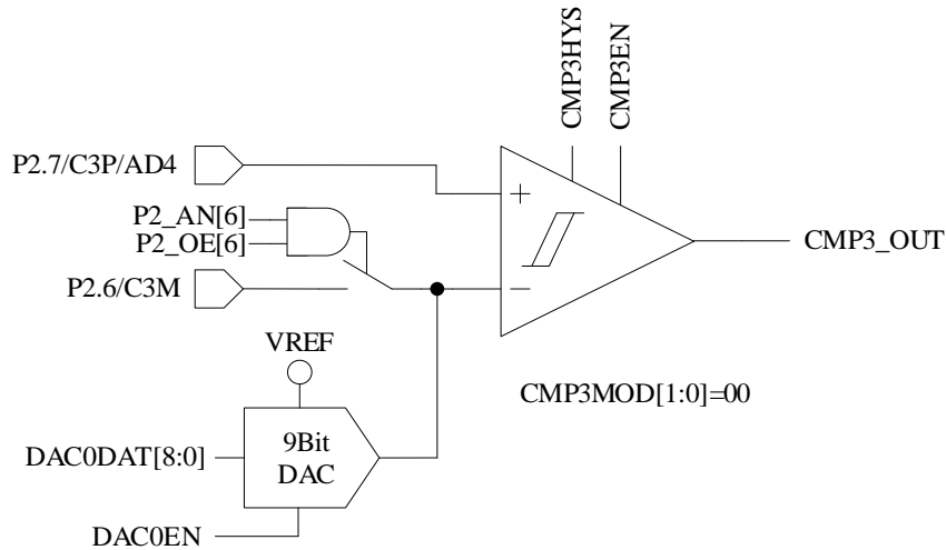
图 28-2 单比较器输入模式
