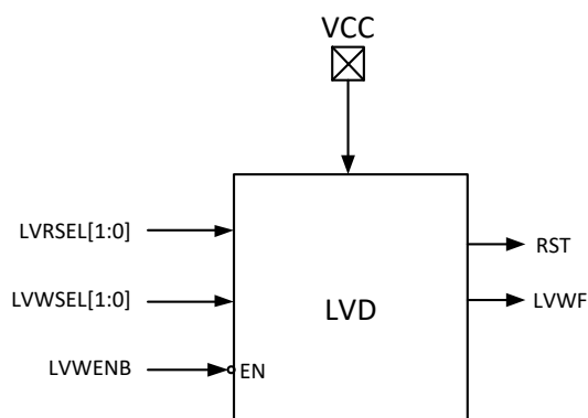
图 29-3 低电压检测模块
