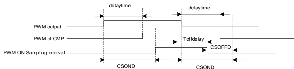
图 28-14 PWM ON 采样模式
