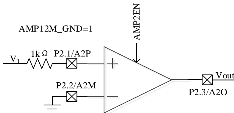
图 27-10 AMP2 工作在 PGA 单端输入模式
