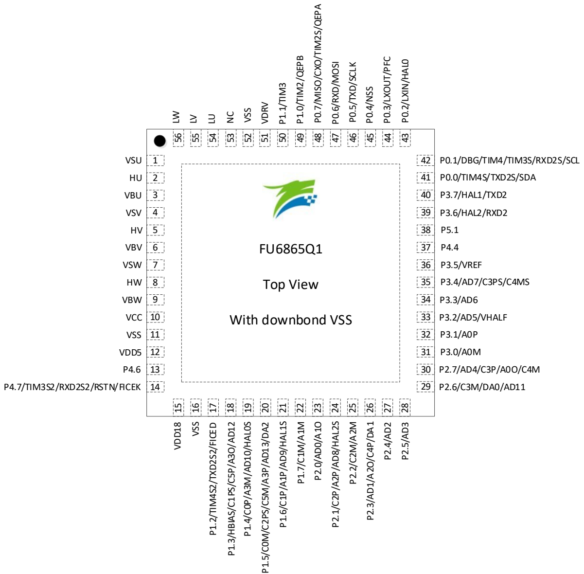
图 2-2 Q1 QFN56 引脚图
