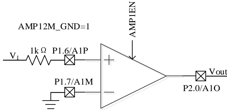
图 27-9 AMP1 工作在 PGA 单端输入模式
