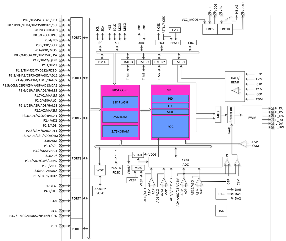
图 1-1 FU6815Q1 功能框图
