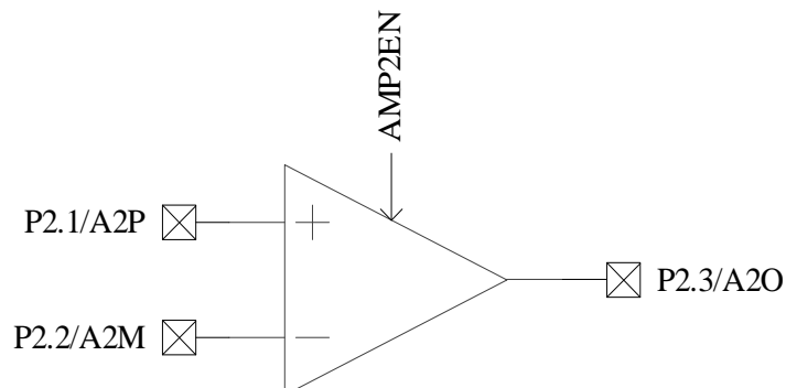
图 27-6 AMP2 输入输出相关端口
