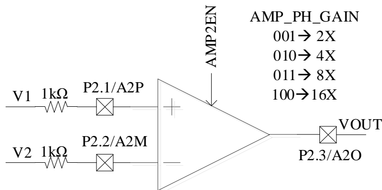
图 27-8 AMP2 工作在 PGA 差分输入模式
