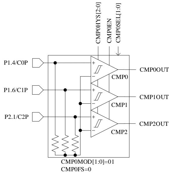
图 28-10 有内置电阻三比较器模式，无功能转移
