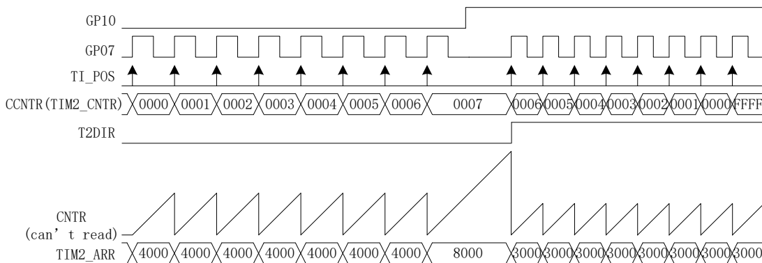
图 15-13 步进模式时序图
