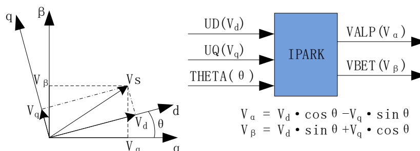
图 13-2 Park 逆变换
