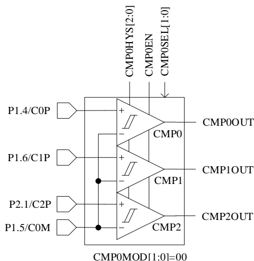
图 28-9 无内置电阻三比较器模式
