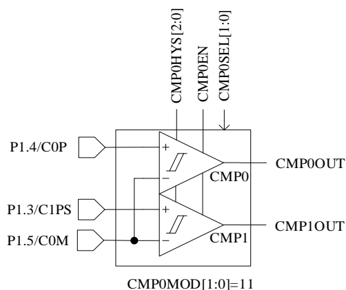
图 28-13 双比较器模式
