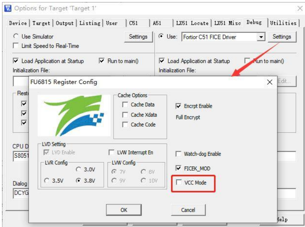
图 29-2 VCC_MODE 配置
