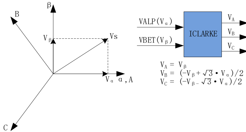
图 13-3 Clarke 逆变换
