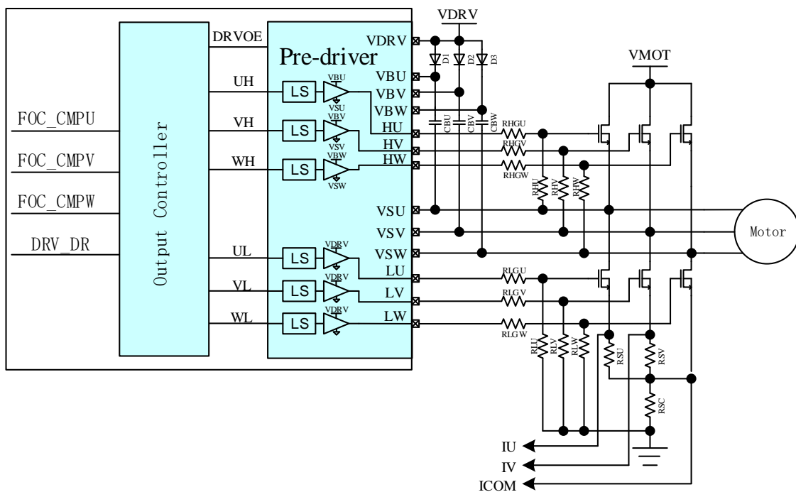
图 18-2 FU6865Q1 Driver 模块框图
