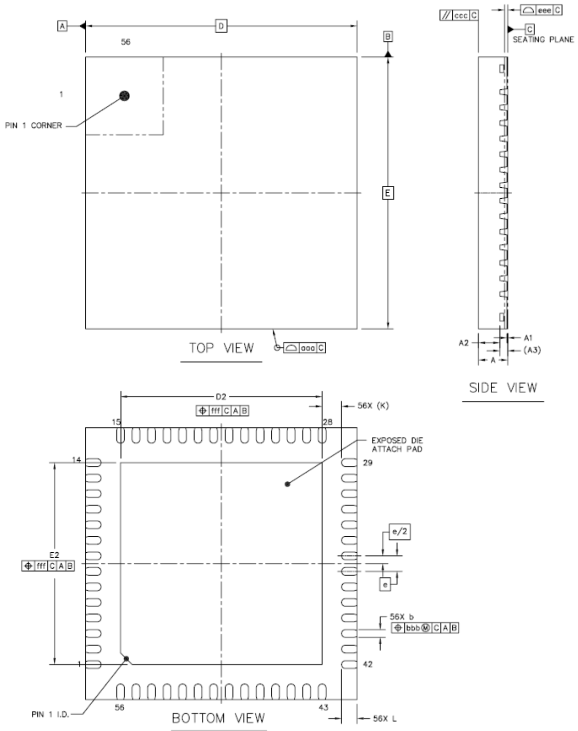
图 3-2 QFN56_7X7 封装尺寸图
