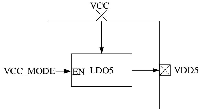
图 29-1 电源模块功能框图
