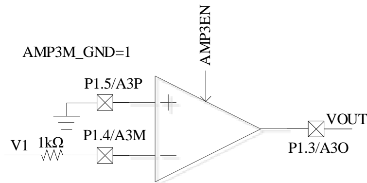
图 27-13 AMP3 工作在 PGA 单端输入模式
