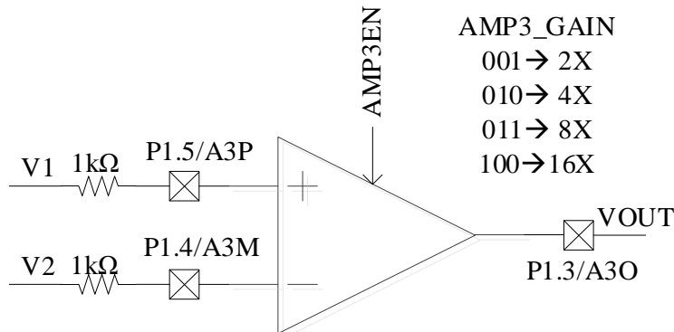
图 27-12 AMP3 工作在 PGA 差分输入模式
