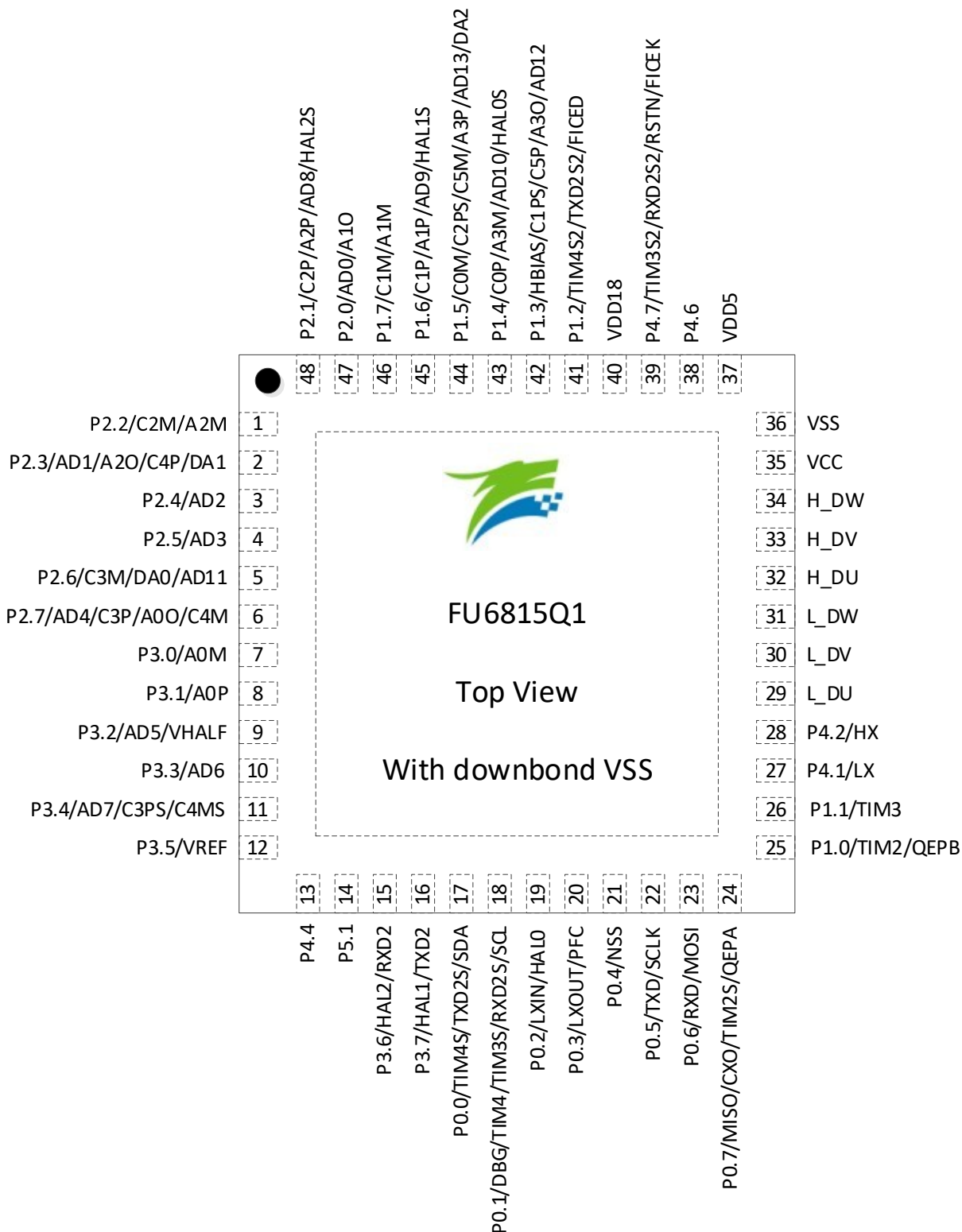
图 2-1 FU6815Q1 QFN48 引脚图
