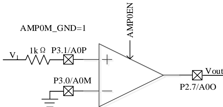
图 27-4 AMP0 工作在 PGA 单端输入模式
