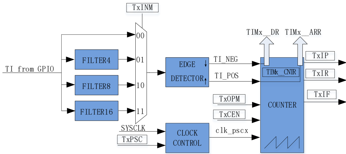
图 16-5 输入捕获模式原理框图
