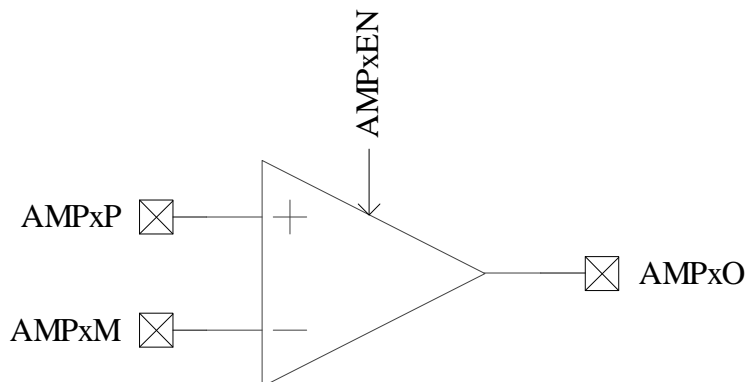
图 27-1 运算放大模块示意图
