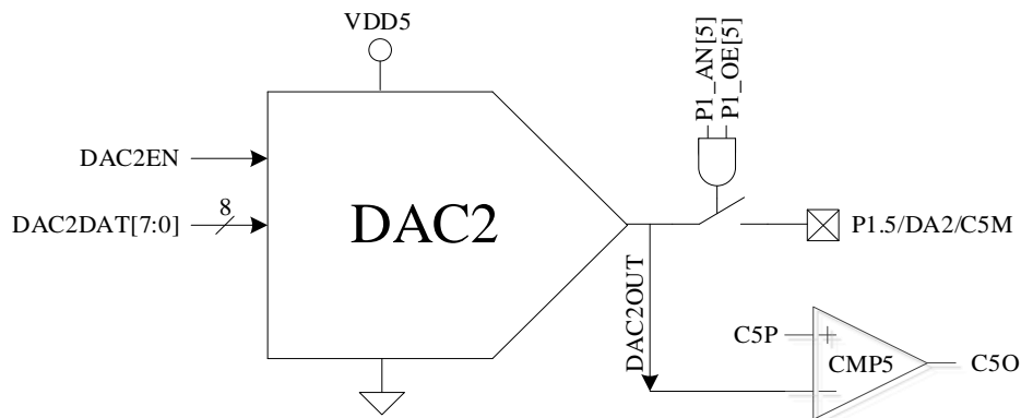
图 23-3 DAC2 功能框图
