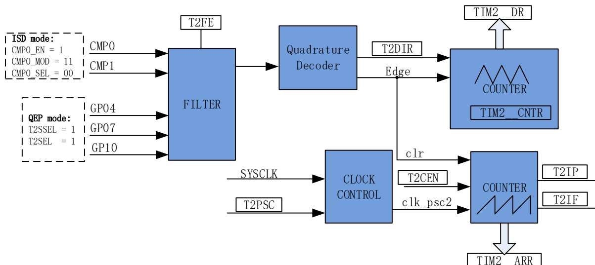
图 15-9 QEP&amp;RSD 模式原理框图
