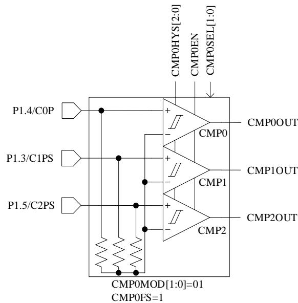
图 28-11 有内置电阻三比较器模式，功能转移
