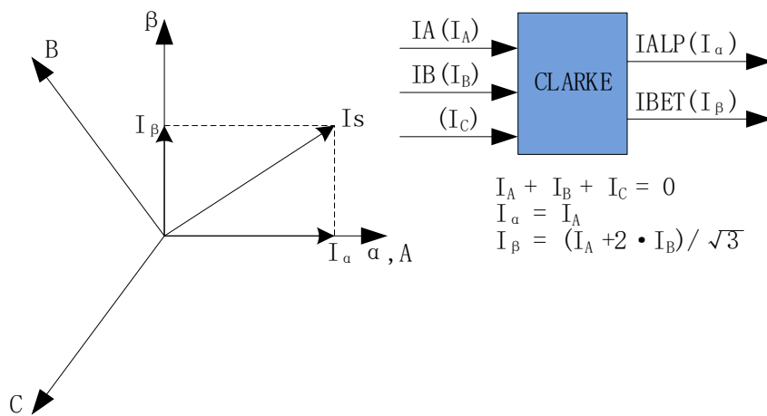
图 13-4 Clarke 变换
