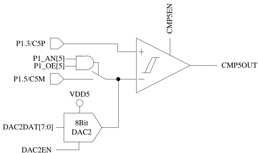
图 28-8 CMP5 模块示意图
