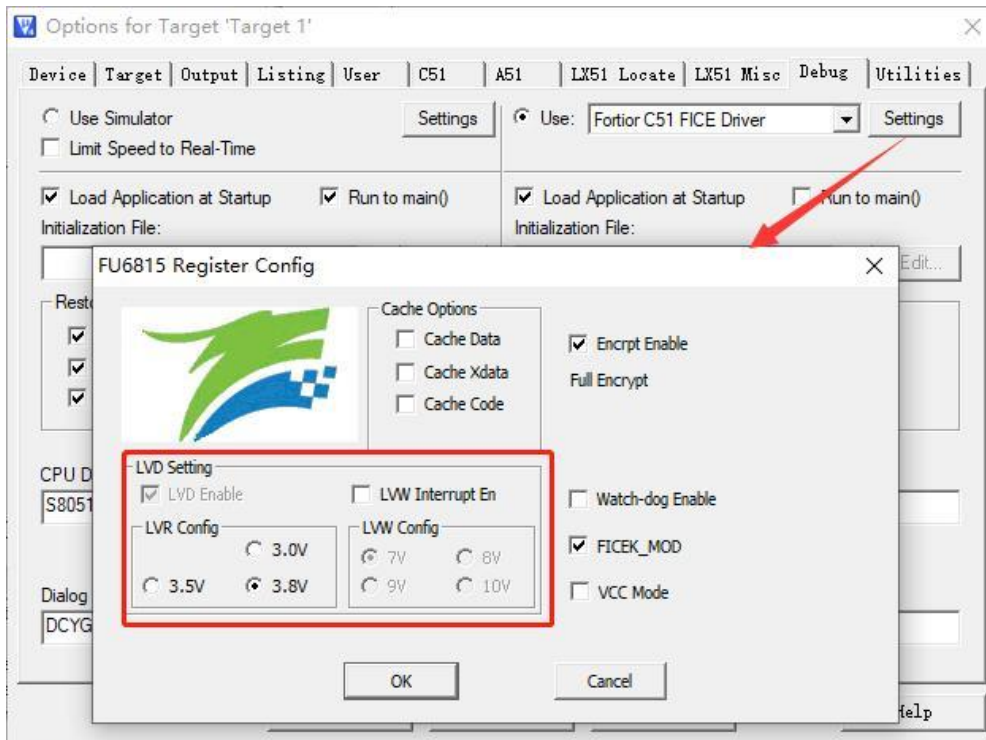
图 29-4 低电压预警电压、中断配置以及低电压复位电压设置
