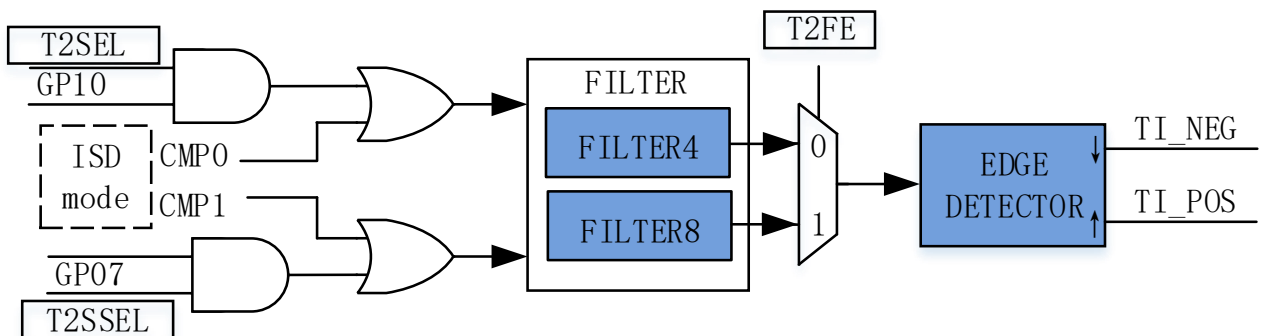
图 15-3 输入信号滤波和边沿检测框图
