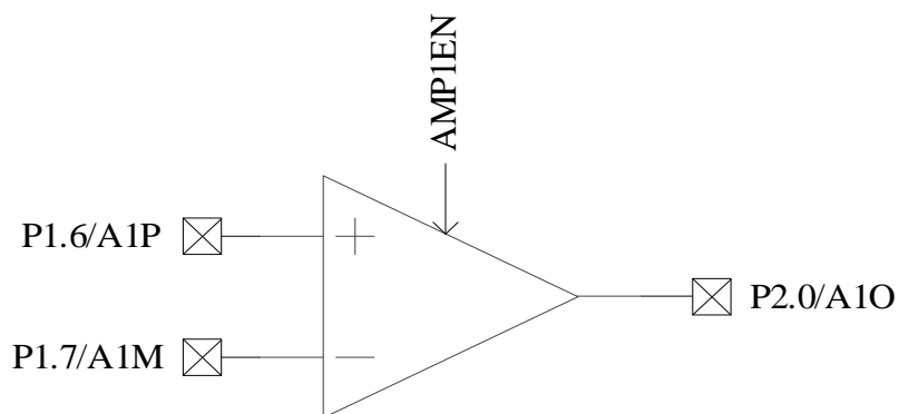
图 27-5 AMP1 输入输出相关端口
