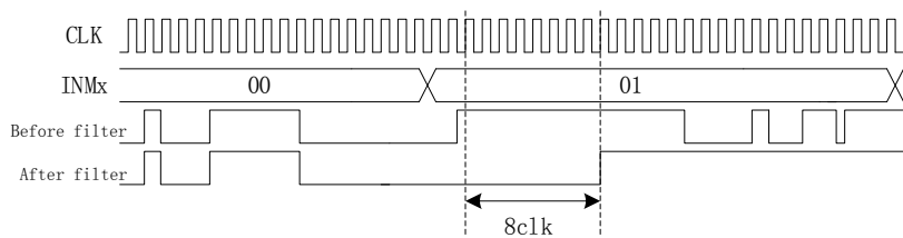
图 15-6 滤波模块时序图
